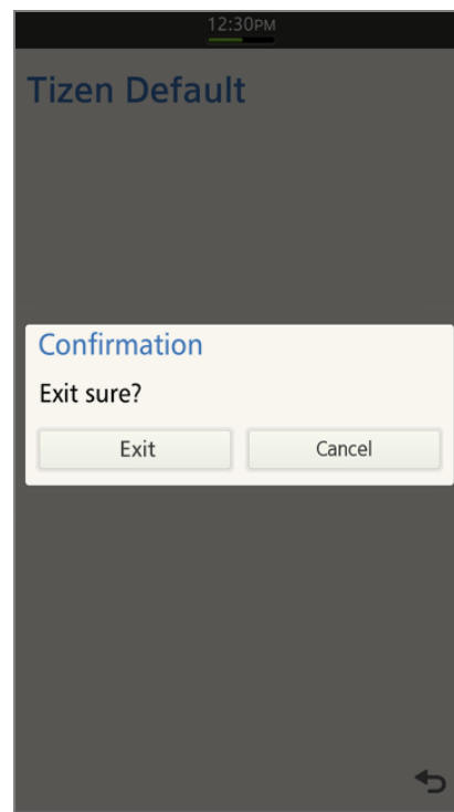
Tizen SDK2.0
