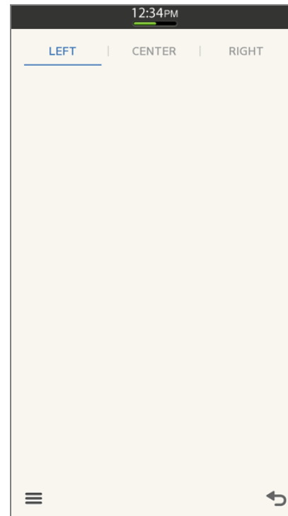
Tizen SDK2.0
