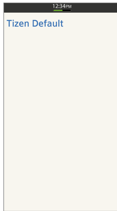
Tizen SDK2.0
