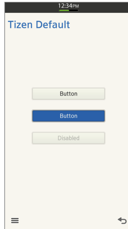
Tizen SDK2.0
